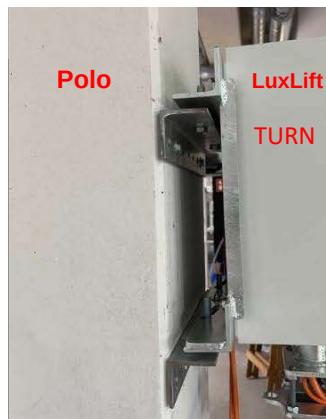
Suspensión de LuxLift TURN
