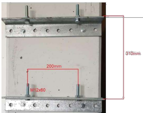
Fijación del soporte Soporte para poste
